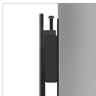
Śruby poziomujące pozwalają na regulację wysokości ekranu
