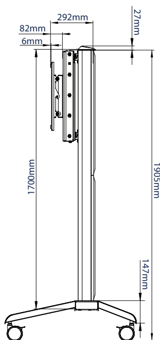
VISTA LATERAL
