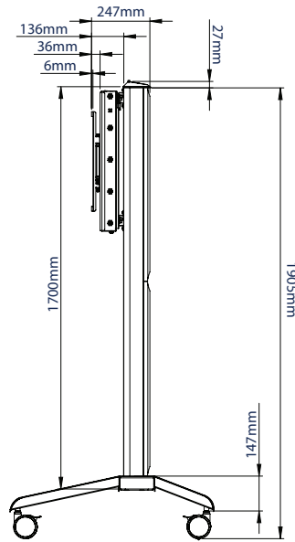
VISTA LATERAL
