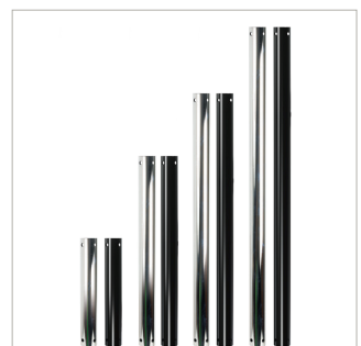
Ø50mm Rohre in dem Längensegment von 0,5 m bis 3 m, ermöglichen das gewünschte Gefälle
