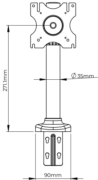
Grommet Clamp
