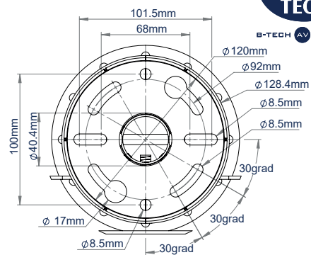
PLACA DE TECHO VISTA SUPERIOR
