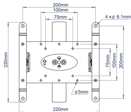
SOPORTE DE MONITOR VISTA FRONTAL
