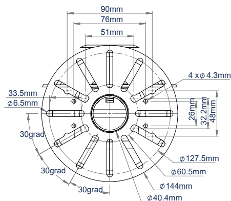
SOPORTE DE CÁMARA CCTV VISTA INFERIOR
