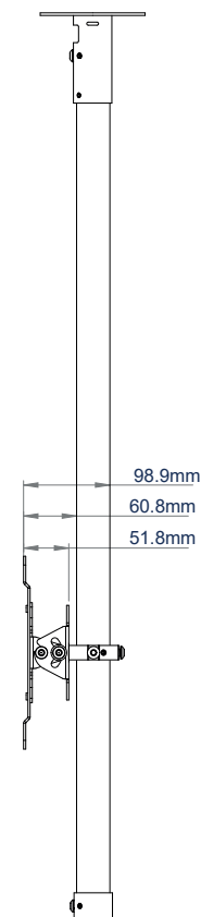
VISTA LATERAL
