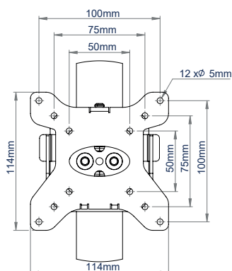
SCHERMBEUGEL VOORAANZICHT
