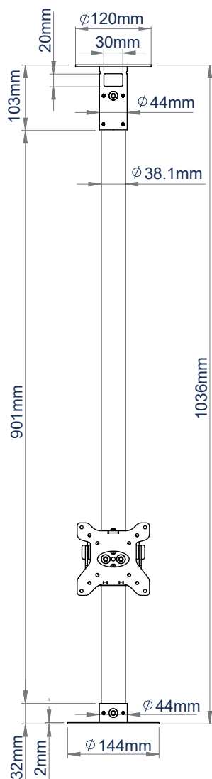
BT5962-FD100 VOORAANZICHT
