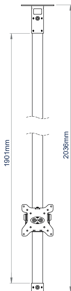
BT5962-FD200 VOORAANZICHT
