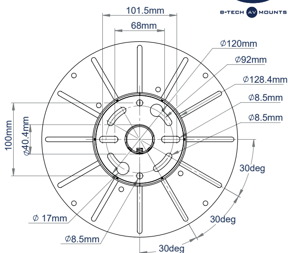
PLAFONDPLAAT BOVENAANZICHT
