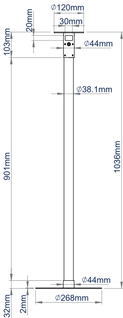
BT5961-FD100 VUE DE FACE
