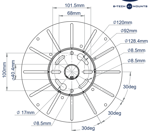
PLAQUE DE PLAFOND VUE DU DESSUS
