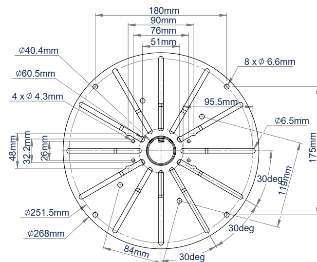
SUPPORT DE CAMÉRA CCTV VUE DE DESSOUS
