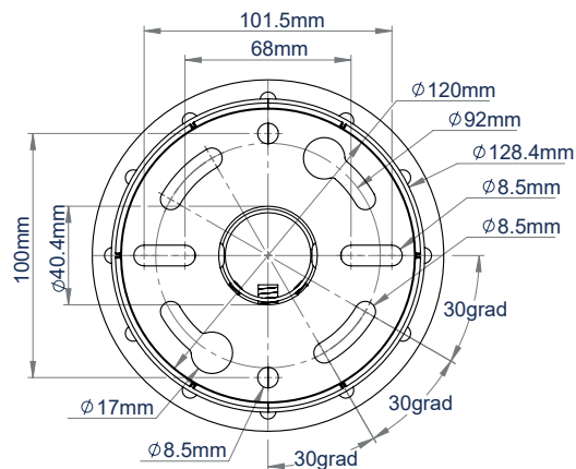
PLACA DE TECHO VISTA SUPERIOR
