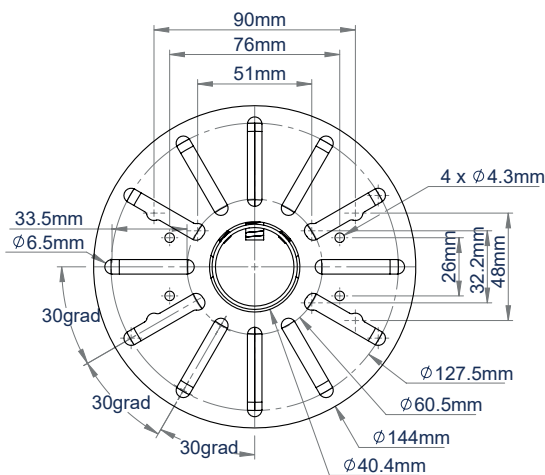
SOPORTE DE CÁMARA CCTV VISTA INFERIOR
