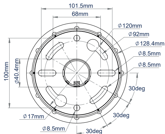
PLAQUE DE PLAFOND VUE DU DESSUS
