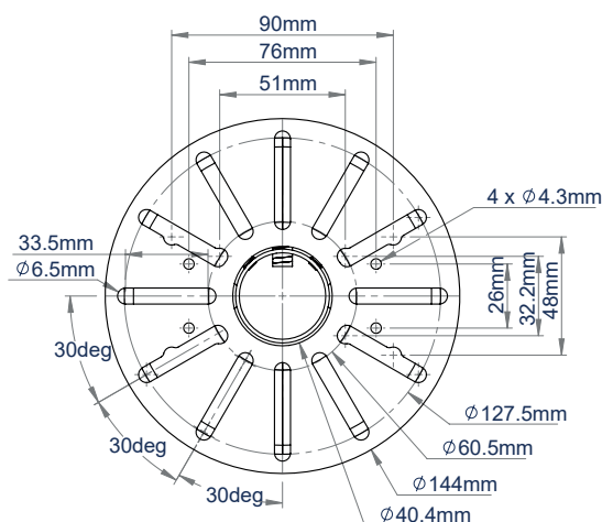
SUPPORT DE CAMÉRA CCTV VUE DE DESSUS
