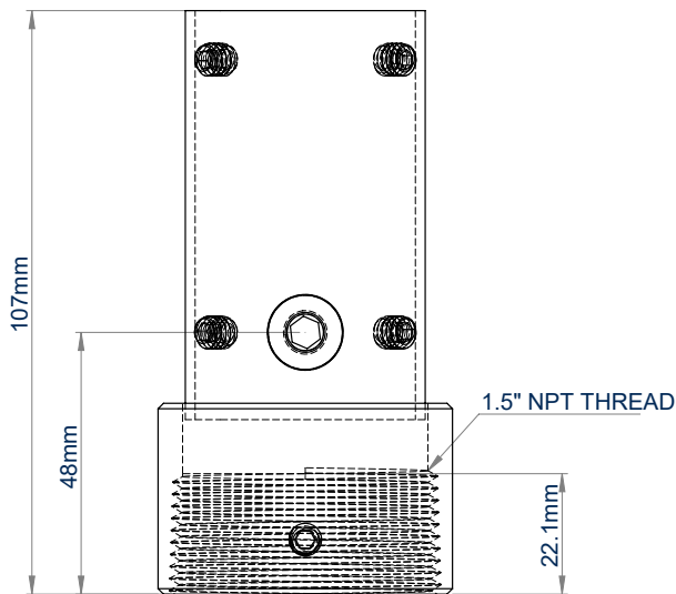
VOORAANZICHT
